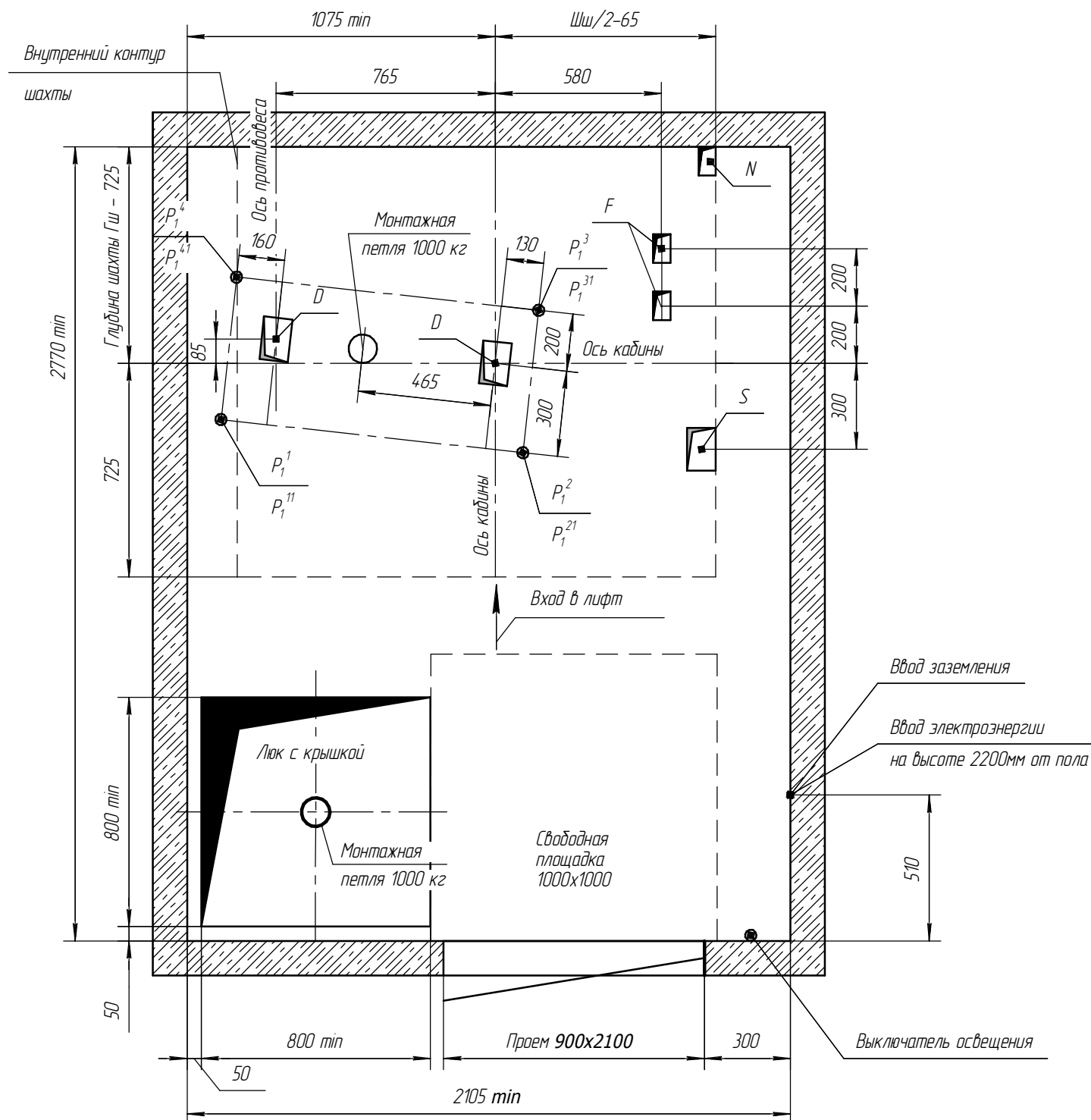
План машинного помещения В-В (1:20) (возможно зеркальное расположение)
