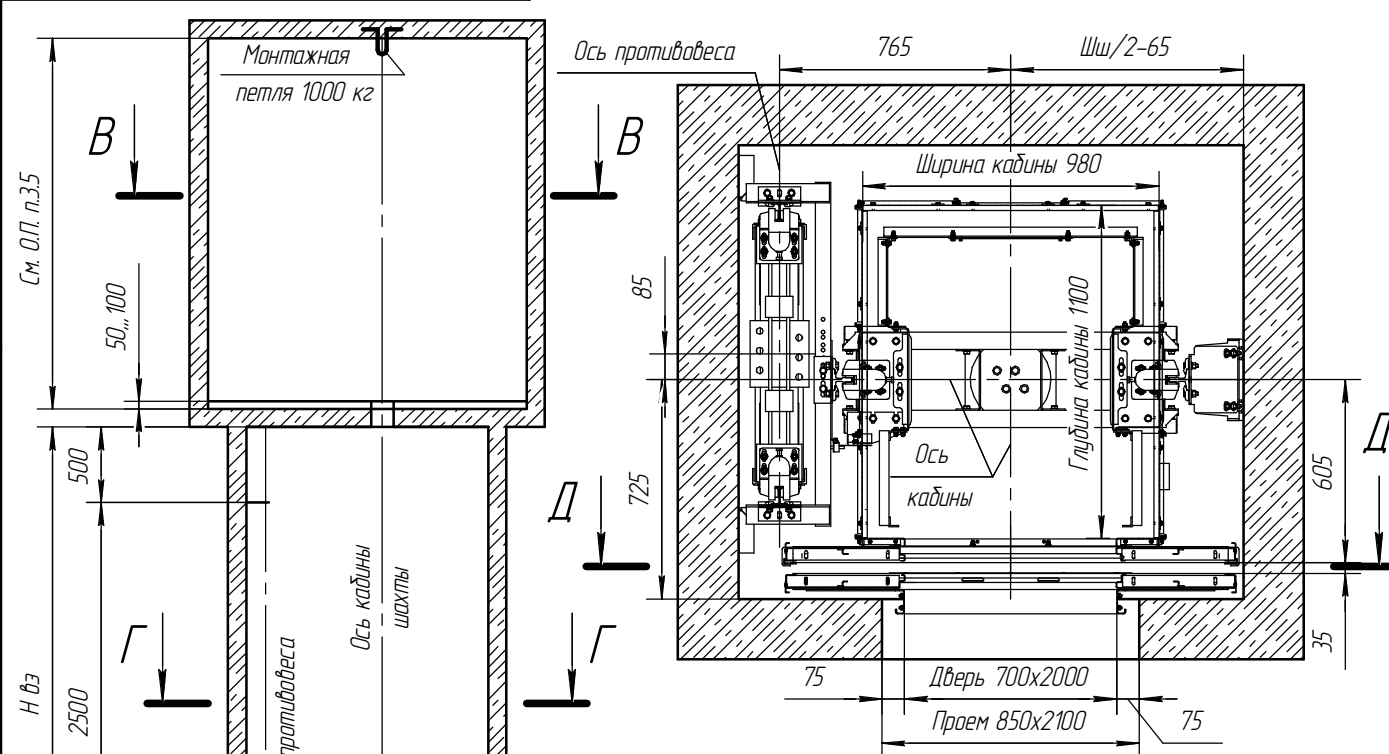
План шахты Г-Г (1:25)
