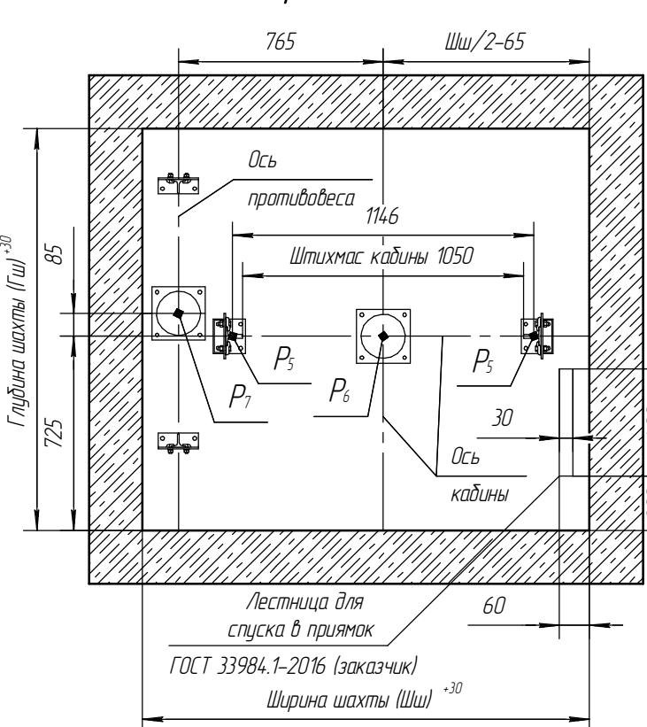
План приямка А-А (1:25)
