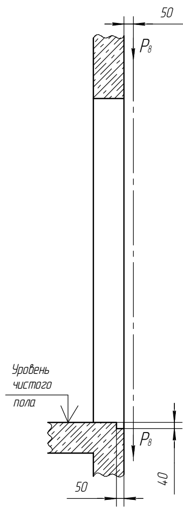
Б-Б (1:15)
